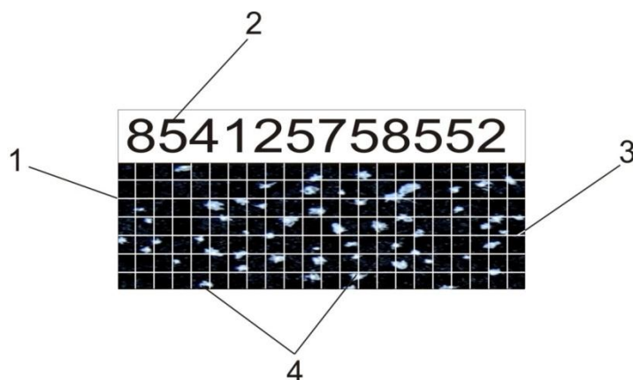
Рис. 7. 1 - невоспроизводимая идентификационная метка, 2 - цифровой код, 3 - информационная сетка, 4 - электроразрядные пятна
