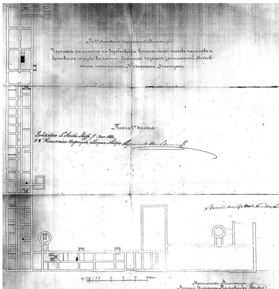
Чертеж к смете на возобновление ветхих печей очагов каминов и дымовых труб в части Красных казарм, занимаемой Московским пехотным юнкерским училищем. План 1-го этажа [32, д. 415, л. 1]
