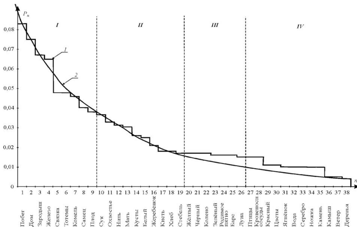
Рис. 1. Гистограмма распределения вероятности различных символов в марийских личных именах (1) и ее аппроксимация показательной функцией (2): область I – главные символы; II – вспомогательные образы-символы; III – дополнительные образы-символы; IV – малоиспользуемые/незначимые образы-символы
